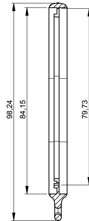
Schnitt A-A
