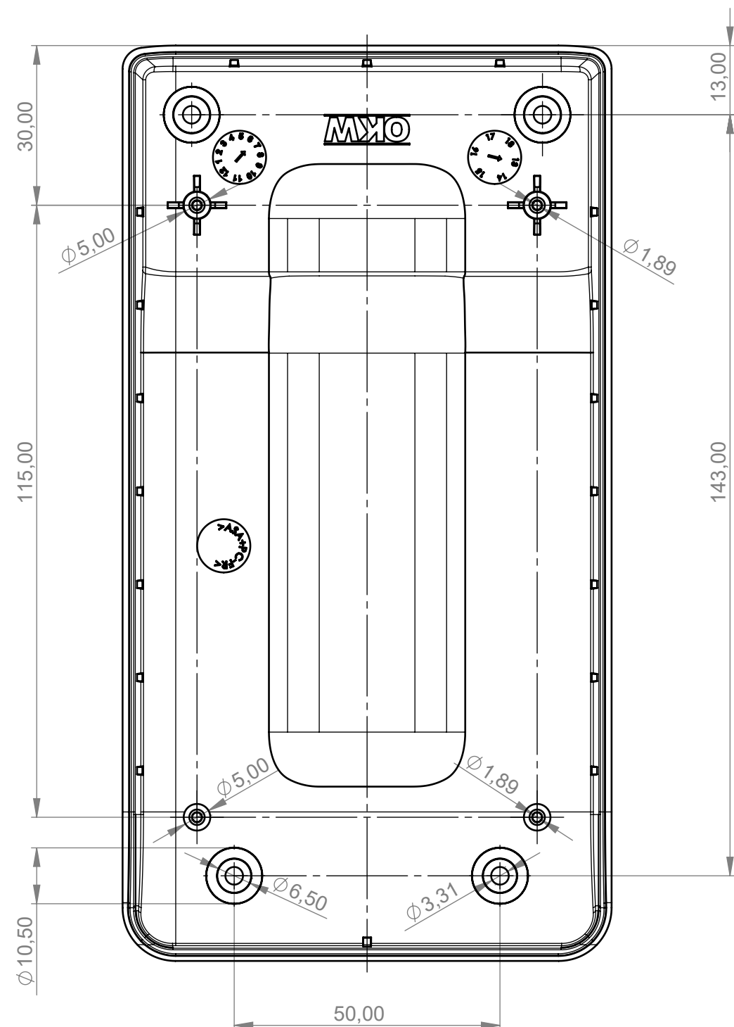
Unterteil Bottom-Part
