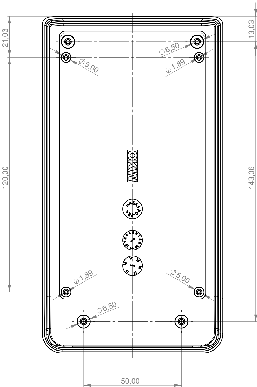
Oberteil Top-Part
