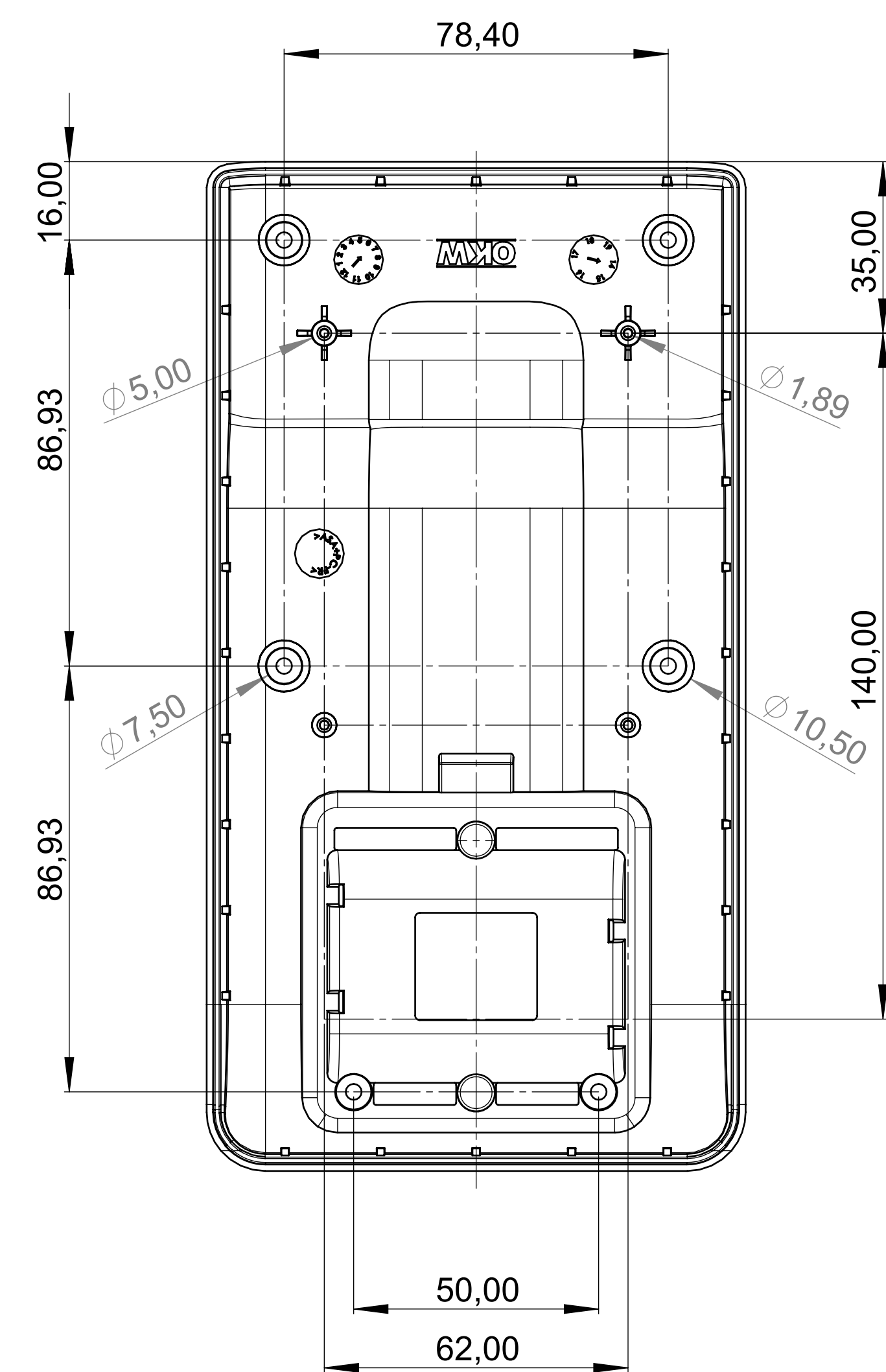
Unterteil Bottom-Part
