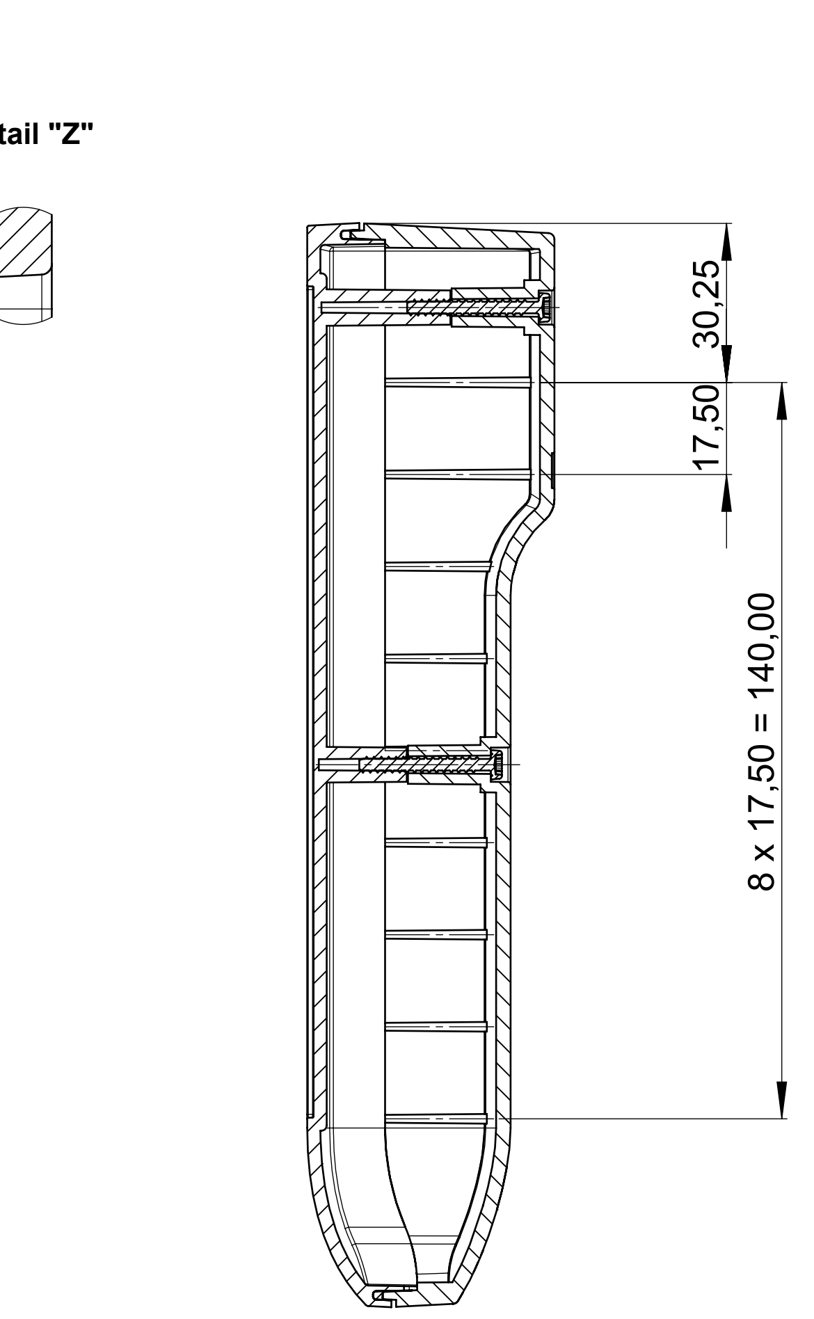
Schnitt B-B Section B-B
