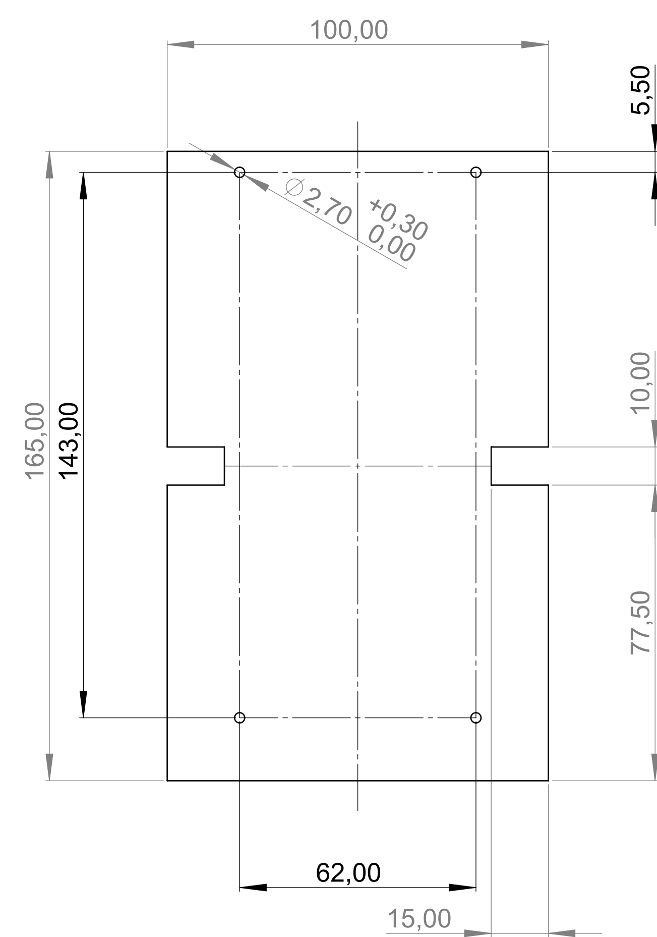
Platine Oberteil P C B Top Part
