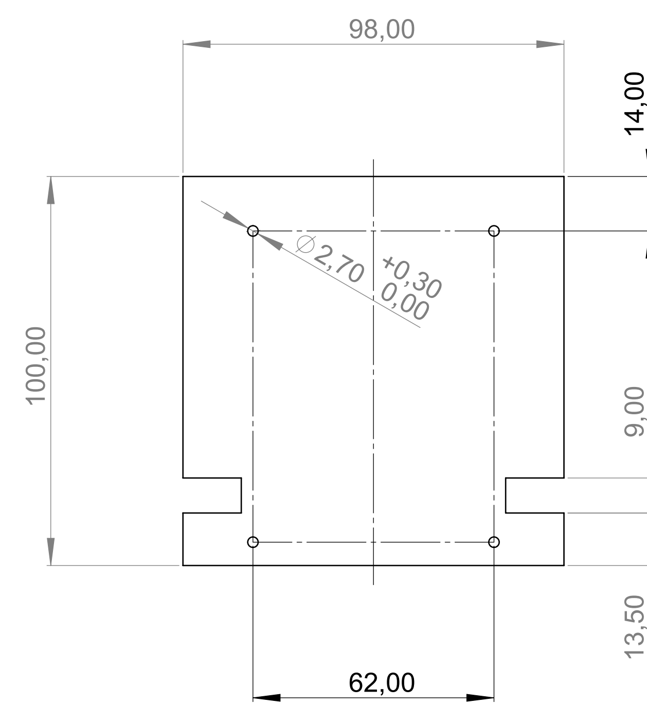
Platine Unterteil P C B Bottom Part
