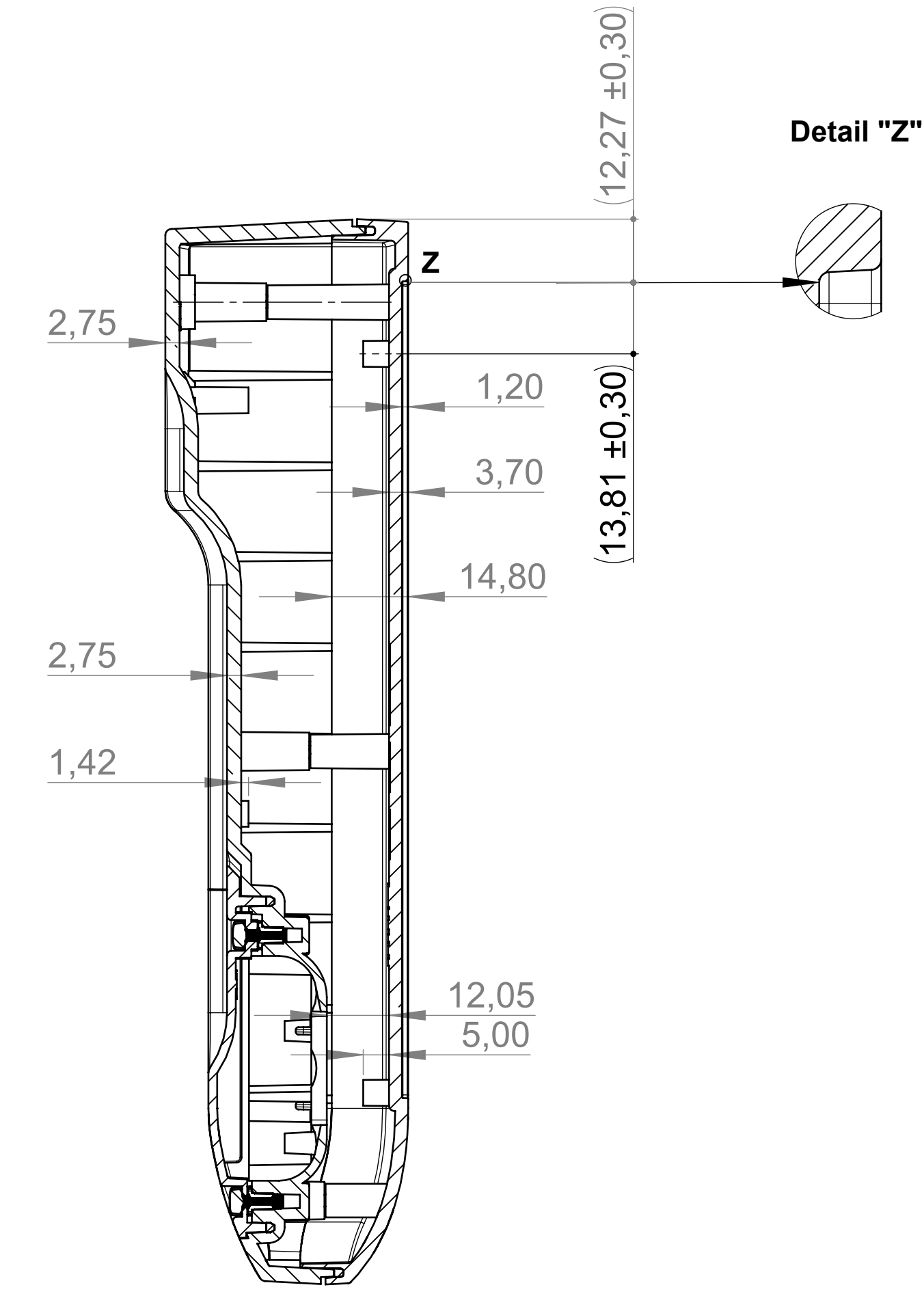
Schnitt A-A Section A-A
