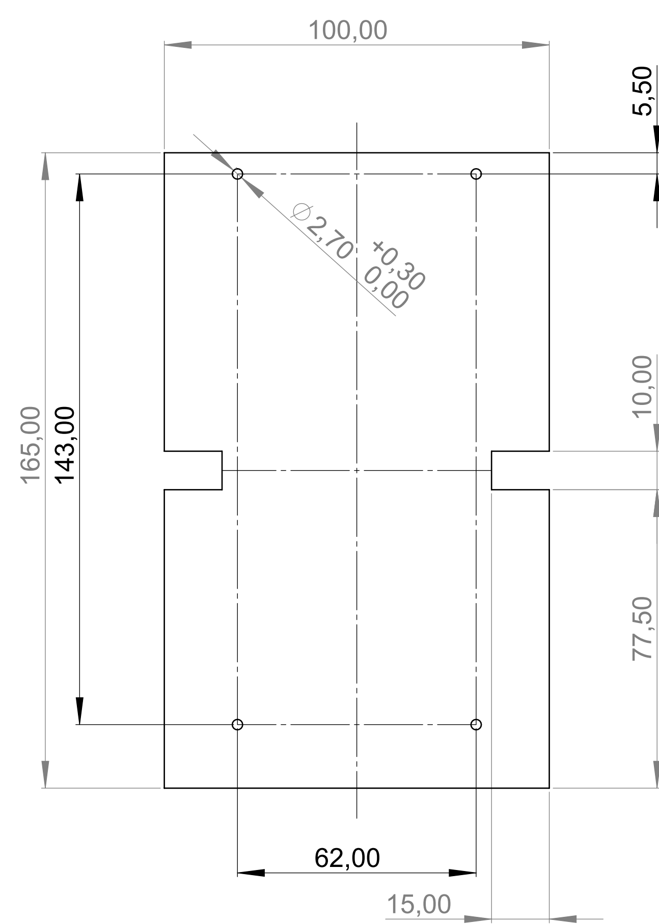
Platine Oberteil P C B Top Part
