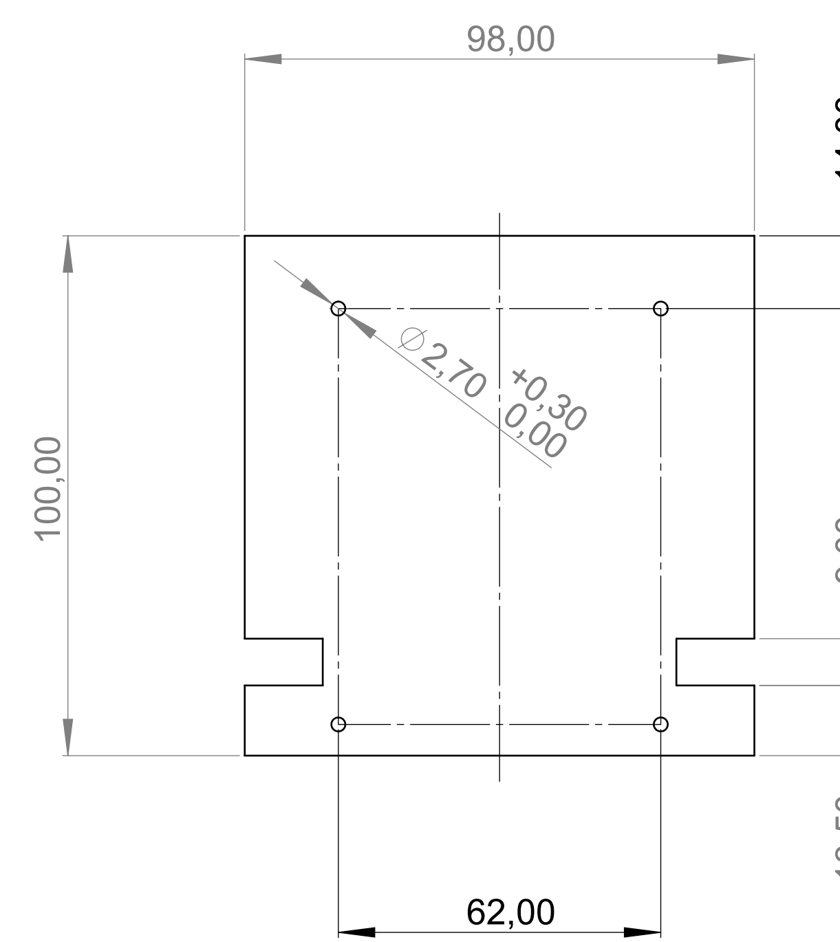
Platine Unterteil P C B Bottom Part
