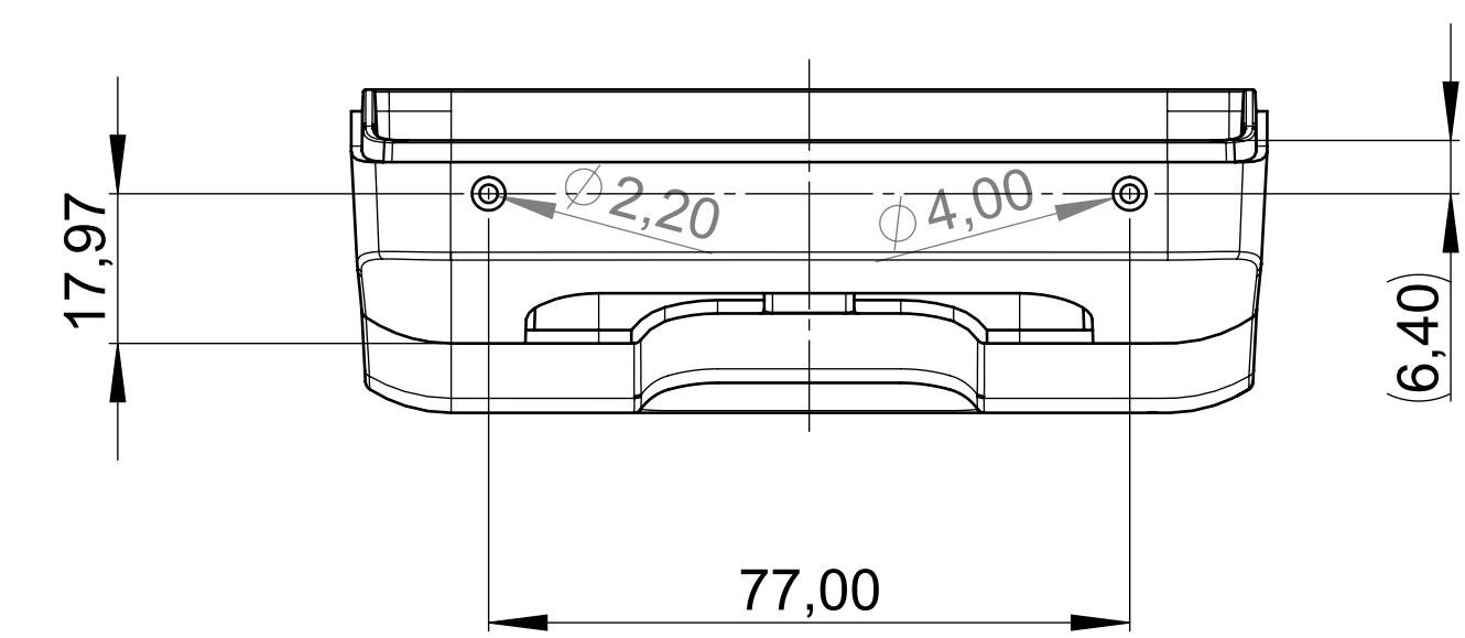
Unterteil Bottom-Part
