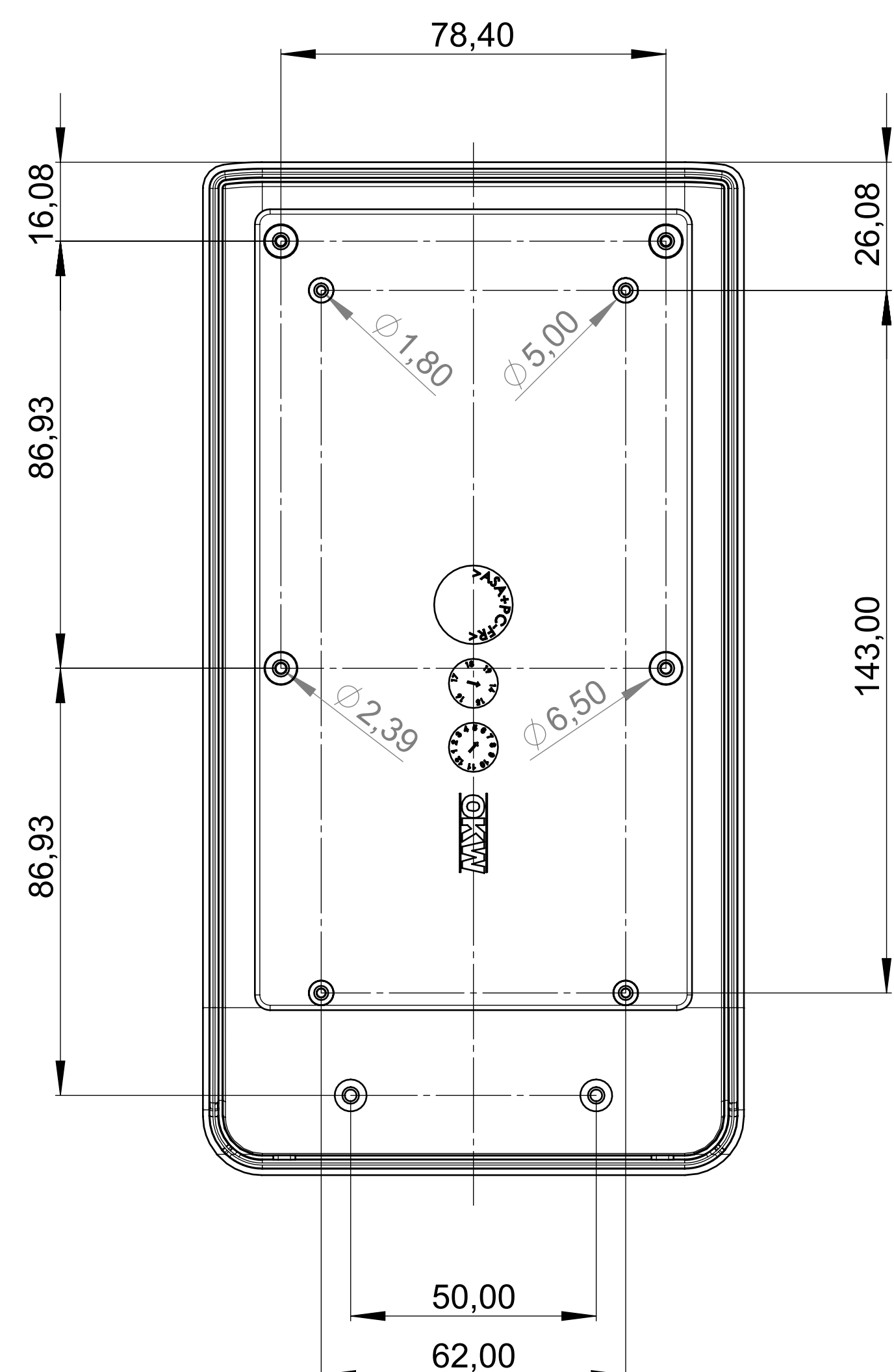
Oberteil Top-Part
