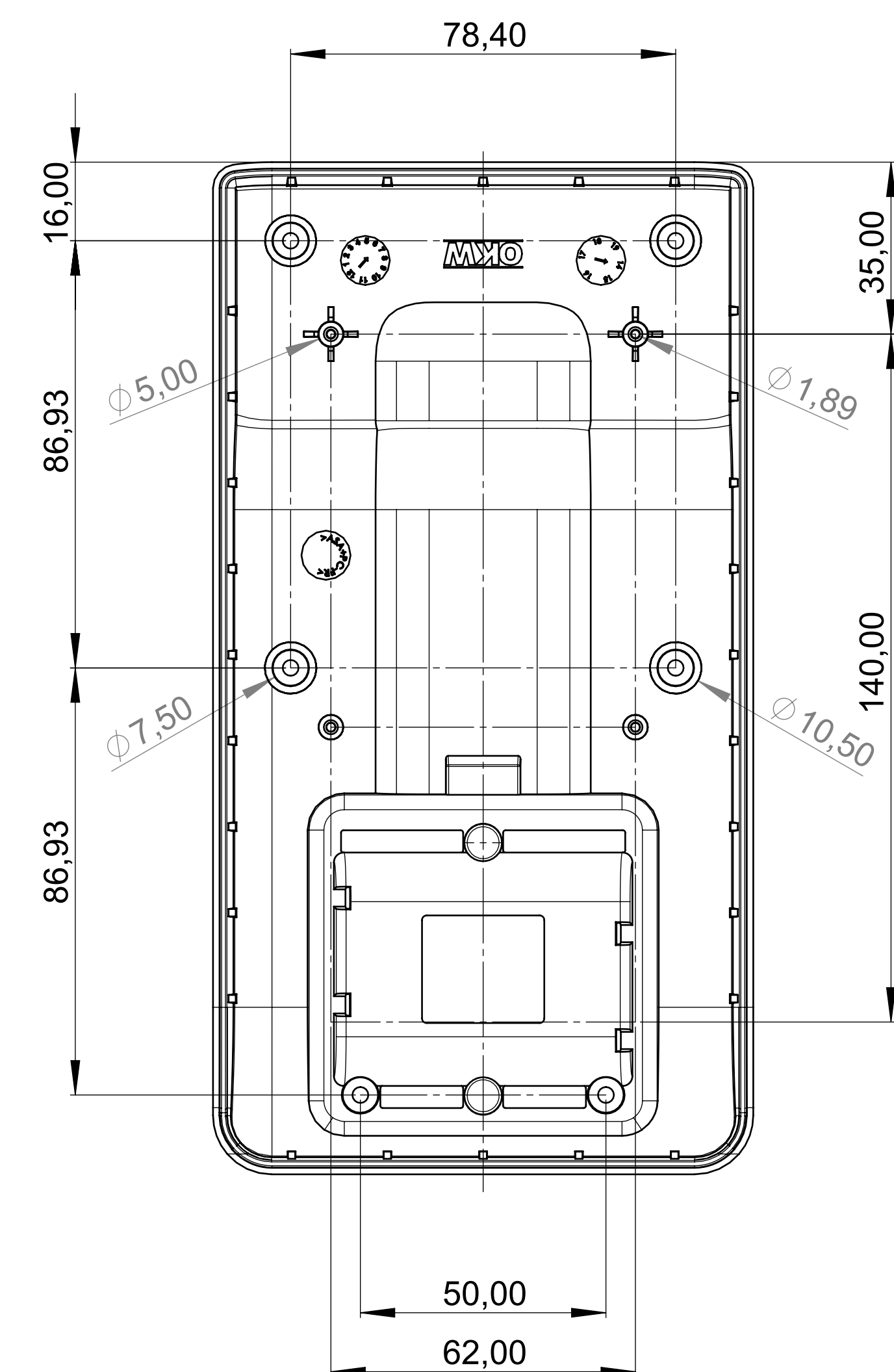
Unterteil Bottom-Part
