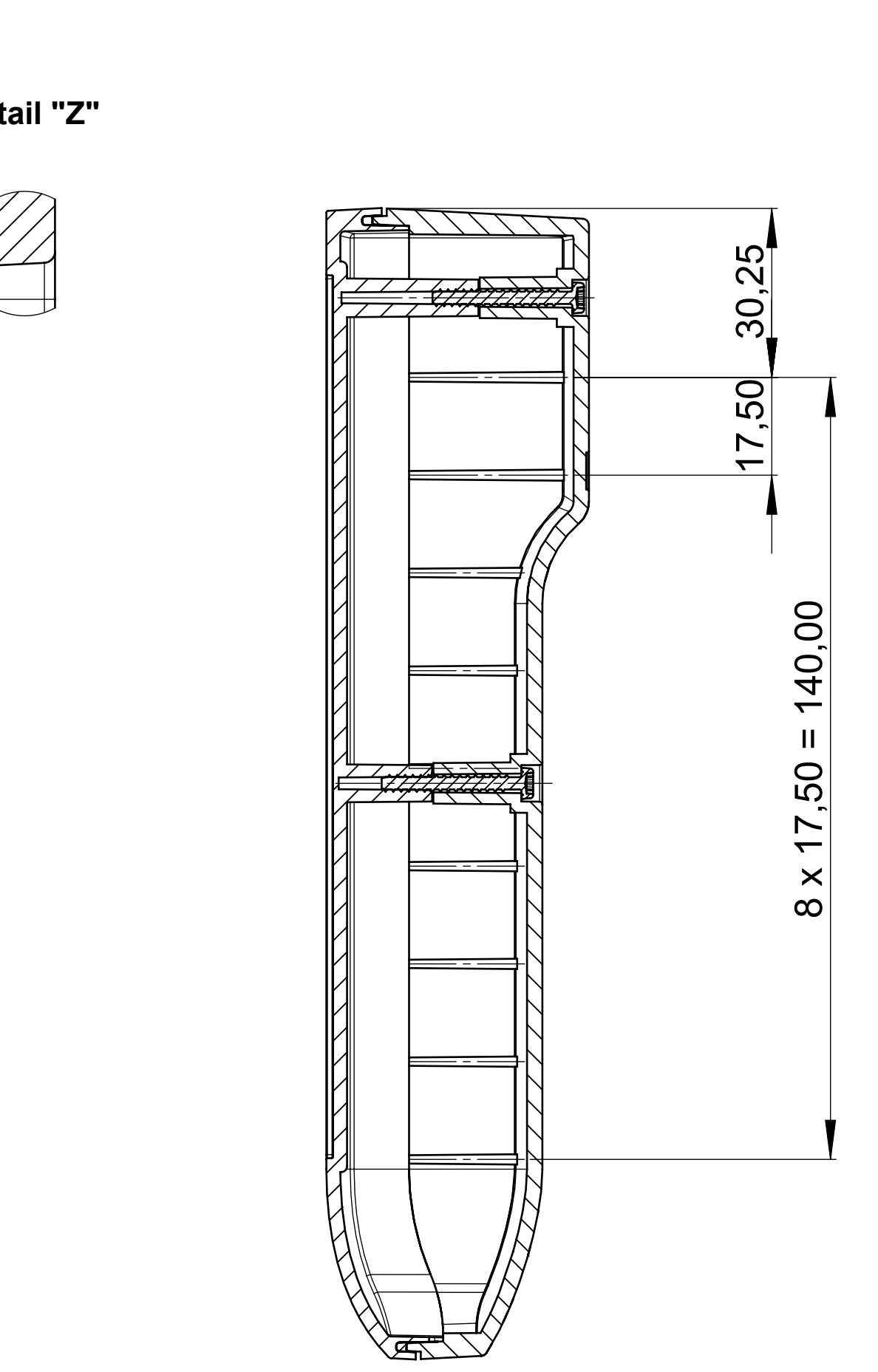
Schnitt B-B Section B-B
