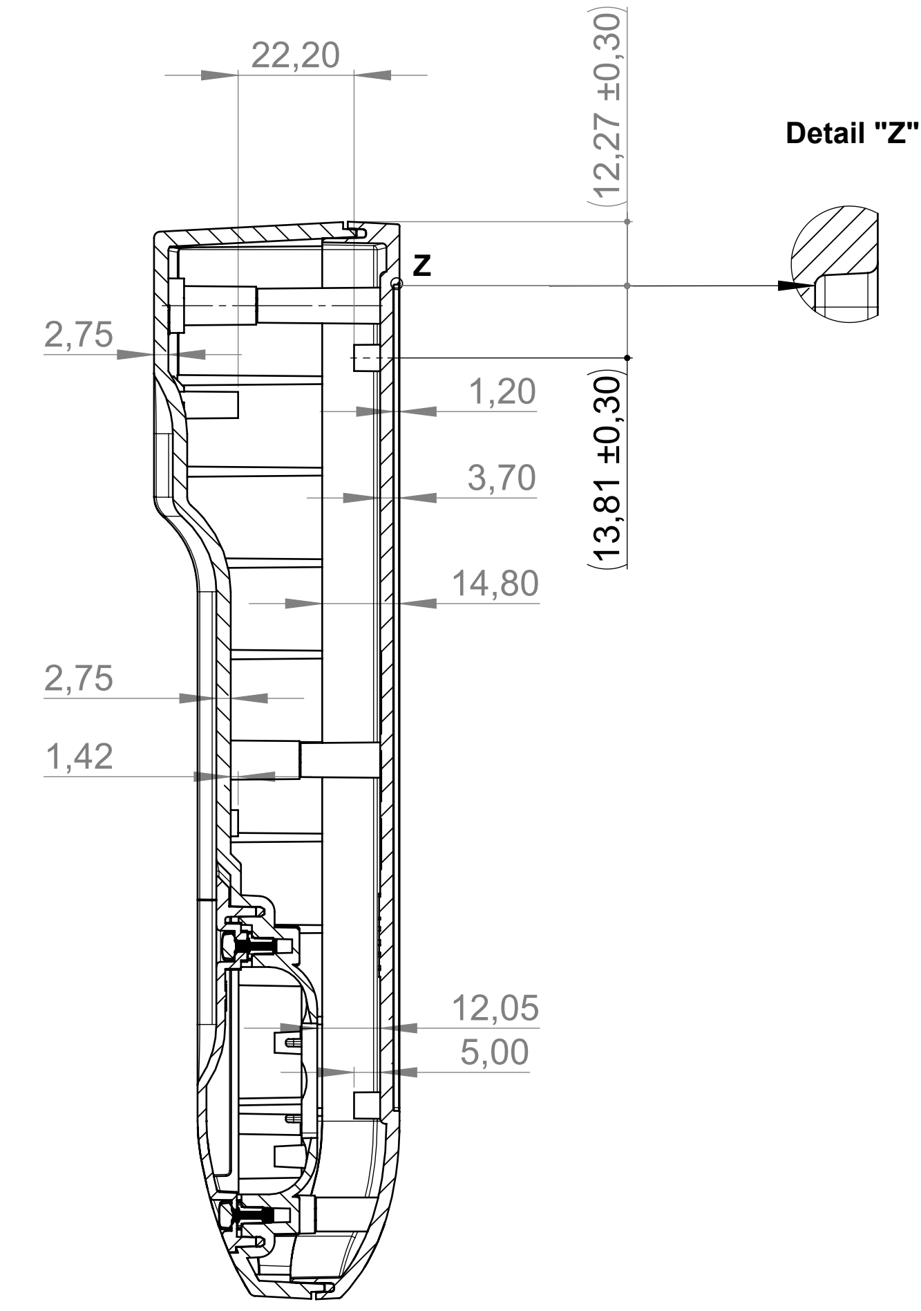
Schnitt A-A Section A-A
