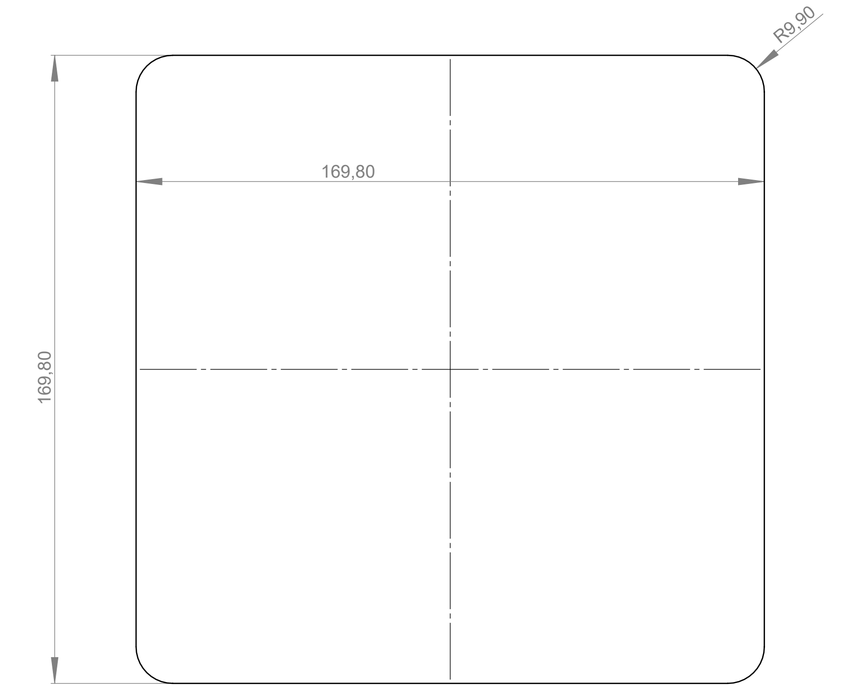
Platine Unterteil P C B Bottom Part
