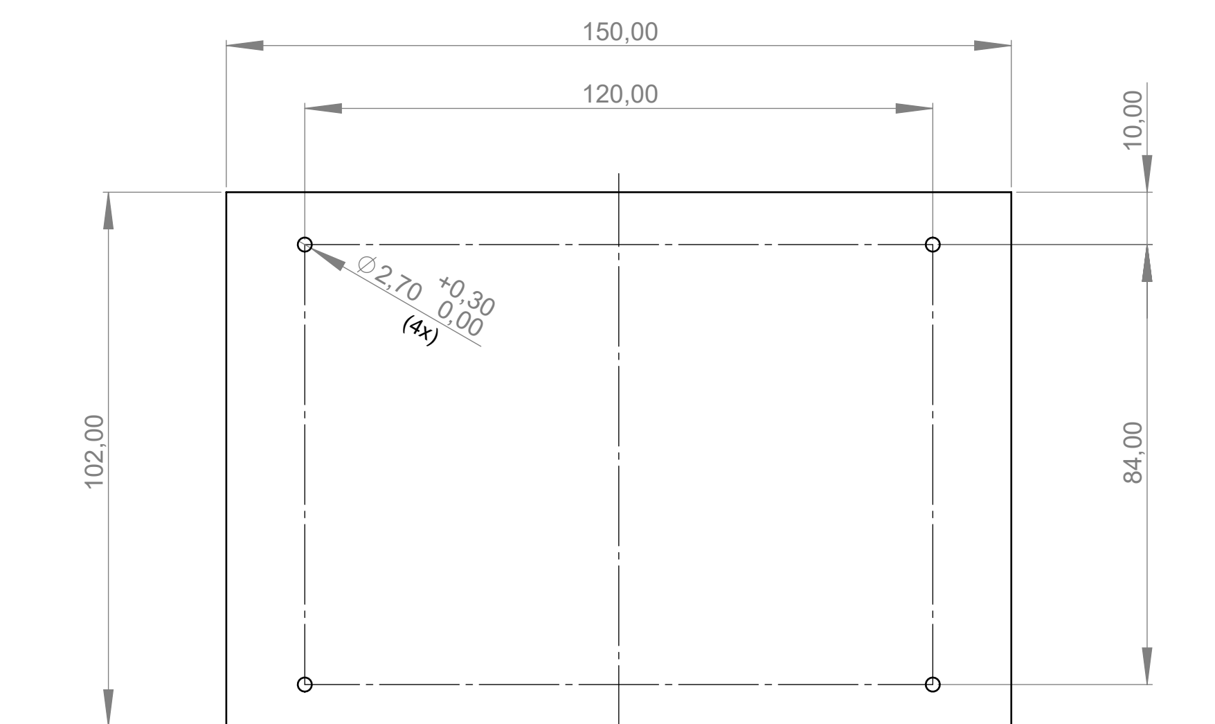
Platine Unterteil P C B Bottom Part
