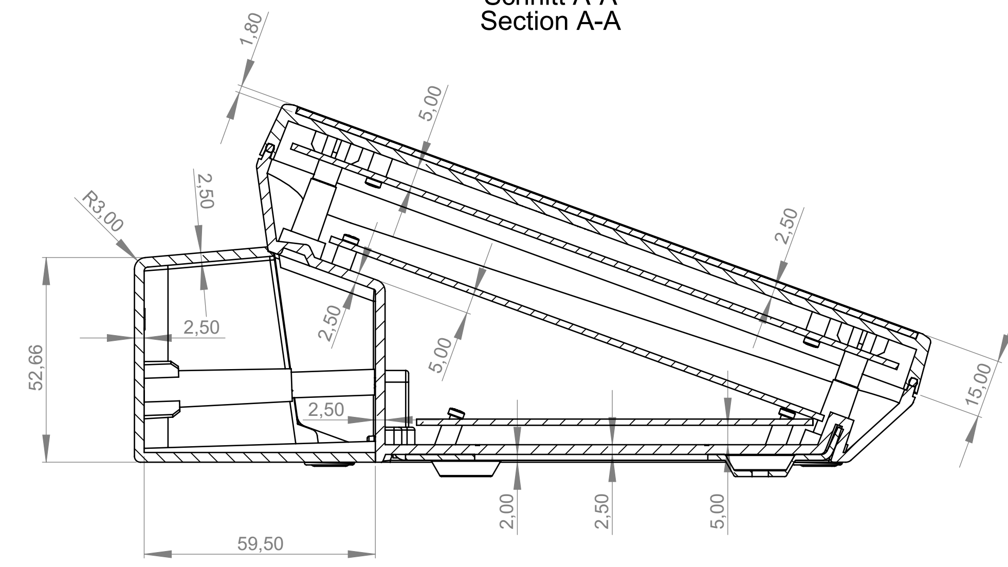
Schnitt A-A Section A-A
