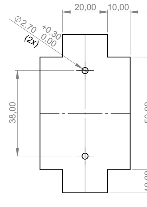
Platine Oberteil P C B Top Part
